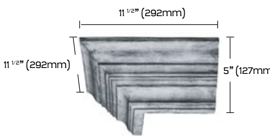
Talon renversé de coin | Corner Box Ogee
