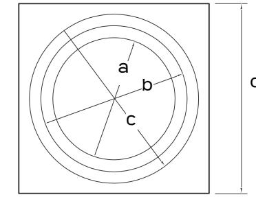
Base de colonne 8" | Column base 8"
