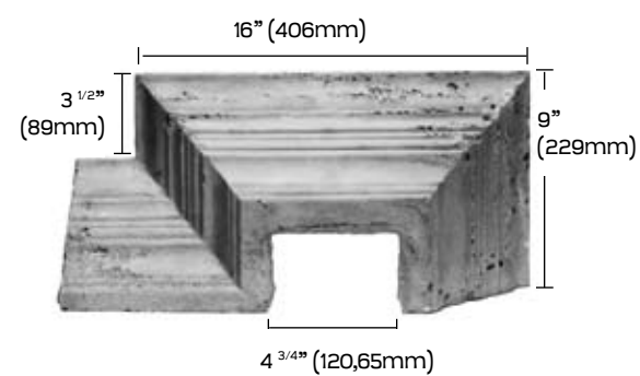
Talon renversé emboîtée | Box Ogee
